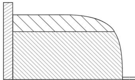
Abb. 4 Querschnitt Schaumbalken Elements®
