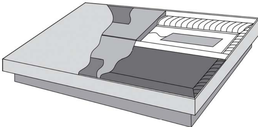
Abb. 8 Vollflächensoftside Elements ®
